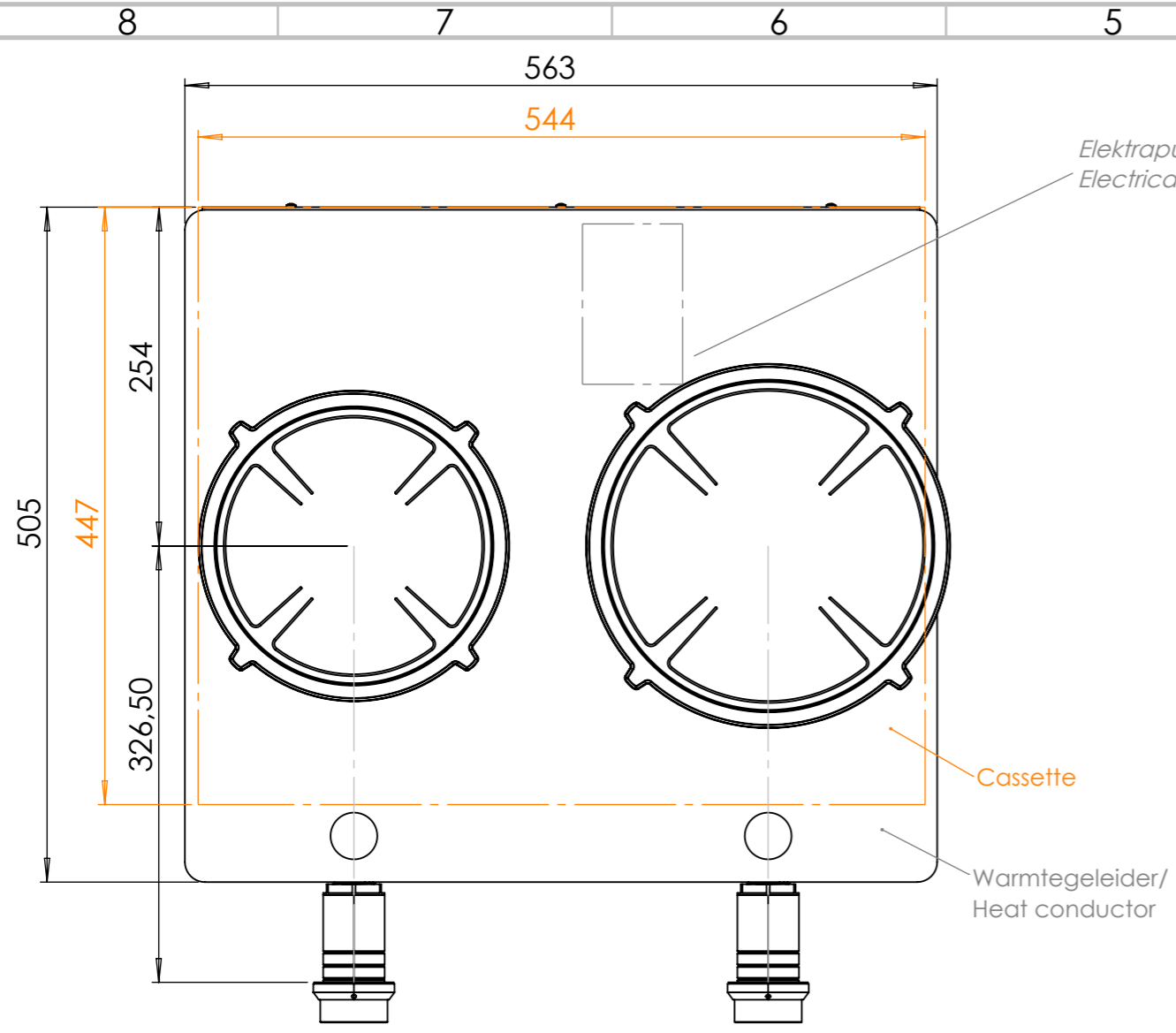
Bovenaanzicht / Top view
