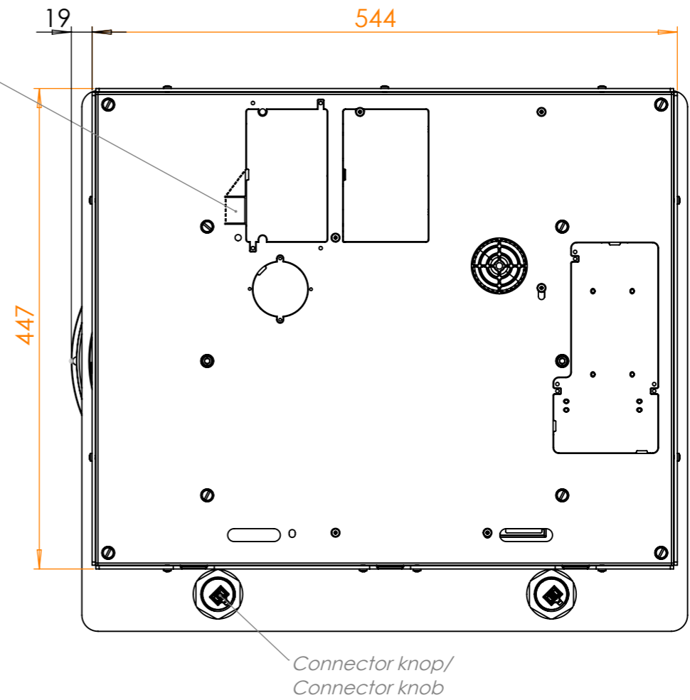
Onderaanzicht / Bottom view
