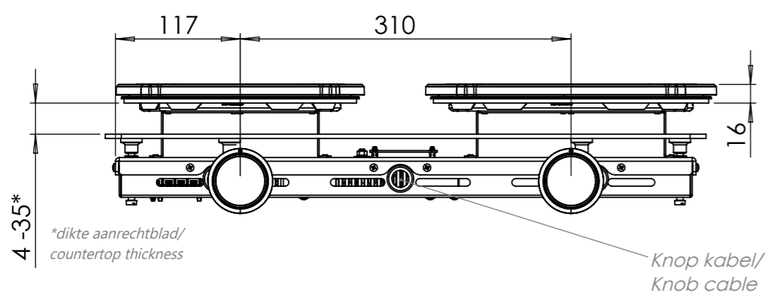
Vooraanzicht / Front view
