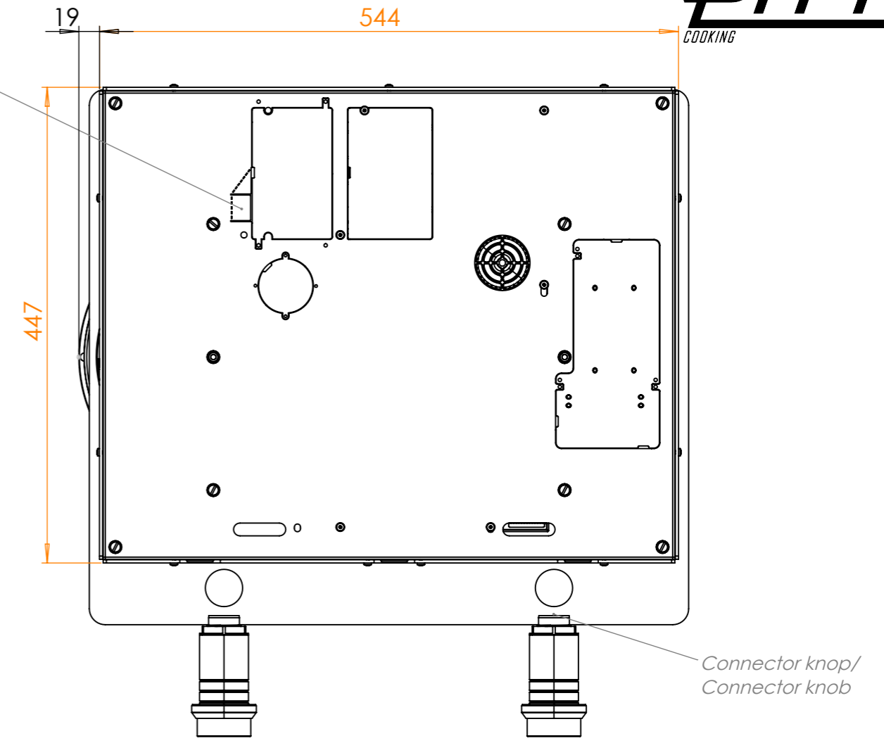
Onderaanzicht / Bottom view
