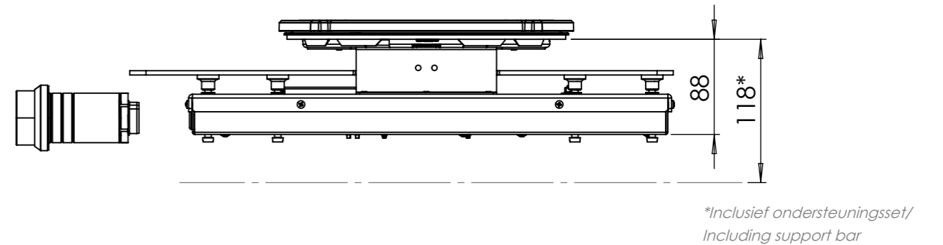
Zijaanzicht / Side view
