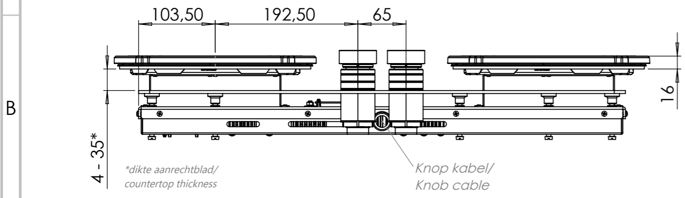
Vooraanzicht / Front view
