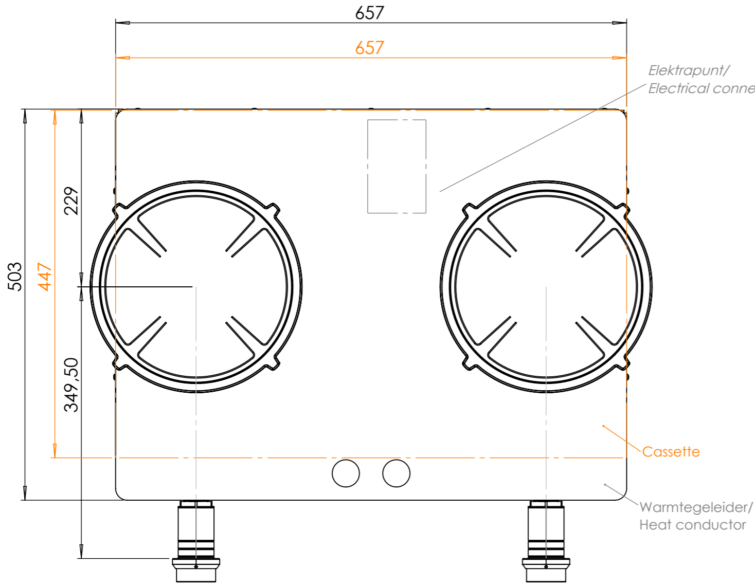
Bovenaanzicht / Top view
