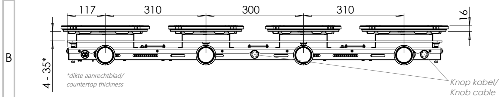
Vooraanzicht / Front view
