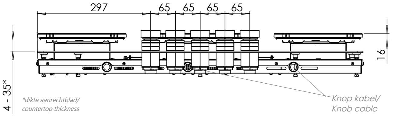
Vooraanzicht / Front view
