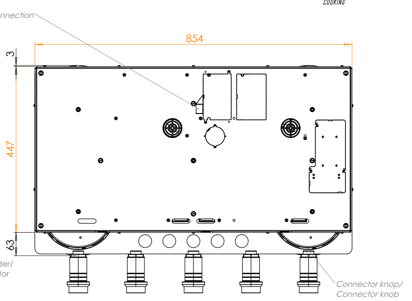
Onderaanzicht / Bottom view
