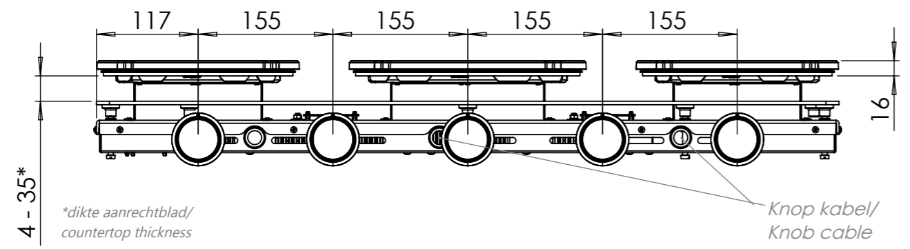
Vooraanzicht / Front view
