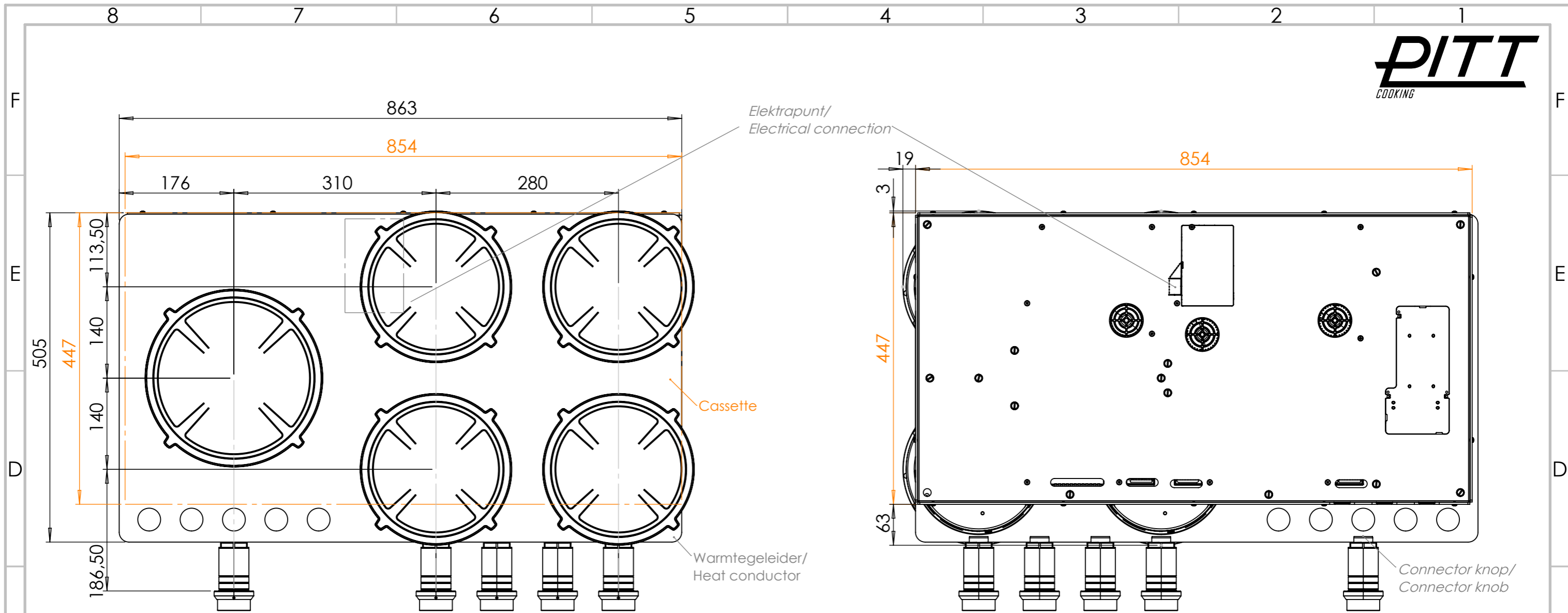
Bovenaanzicht / Top view
