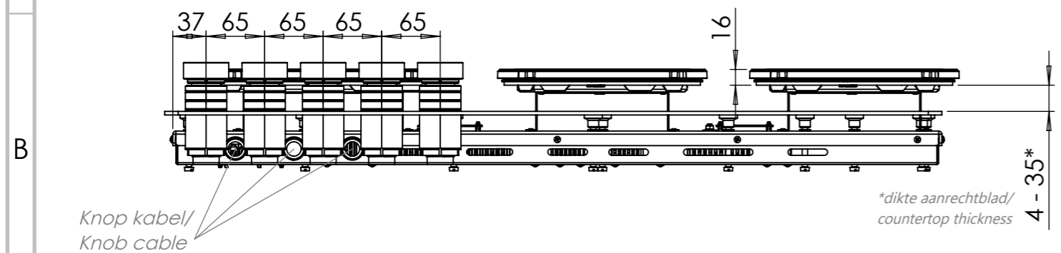
Vooraanzicht / Front view
